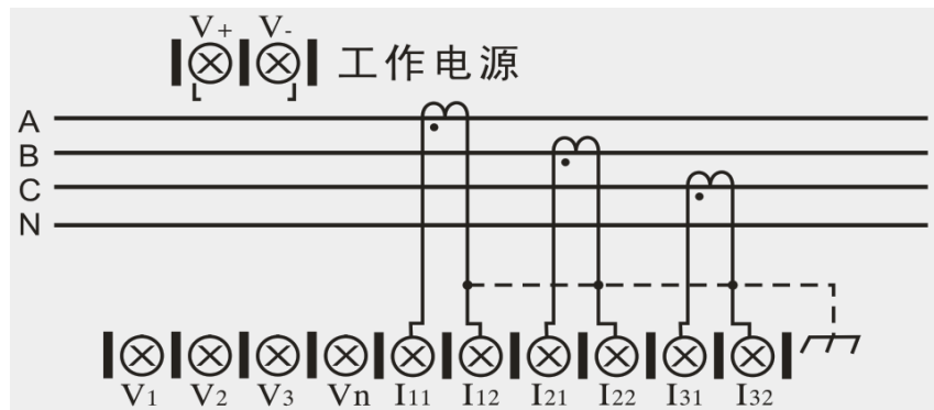
图 5.3 三相四线接线图
