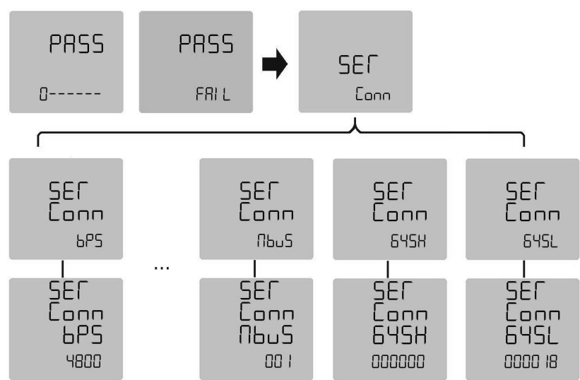
图 4.2 按键设参示意图
