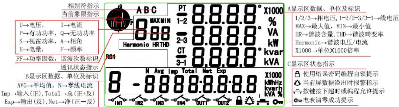
图 4.1 液晶全屏显示说明
