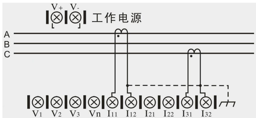
图 5.4 三相三线接线图
