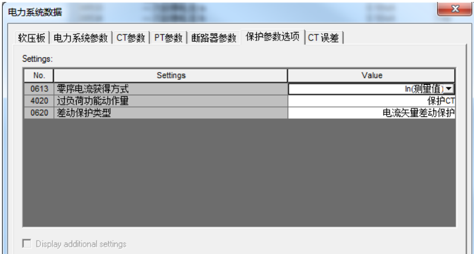
图 1 差动保护类型切换
