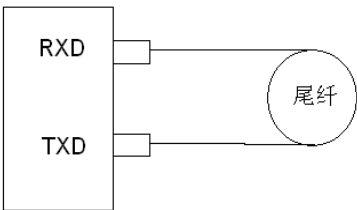
图 5 尾纤连接示意图
